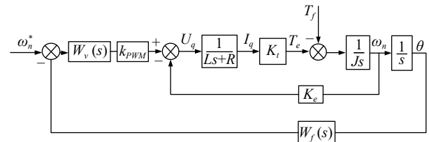
图 2 望远镜速度环数学模型
