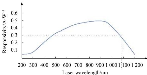
图 4 APD 激光响应度和激光波长关系图 ( M=1 )
