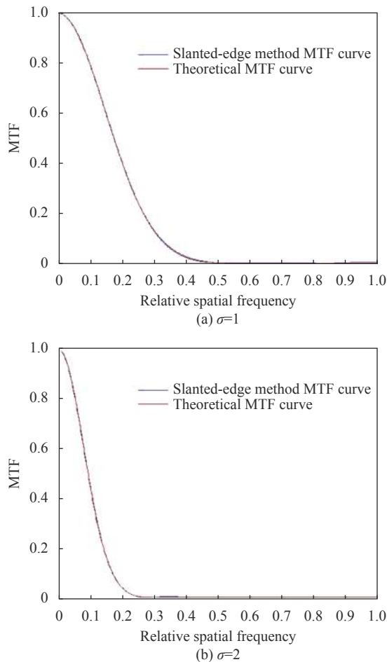
图2 MTF曲线对比
