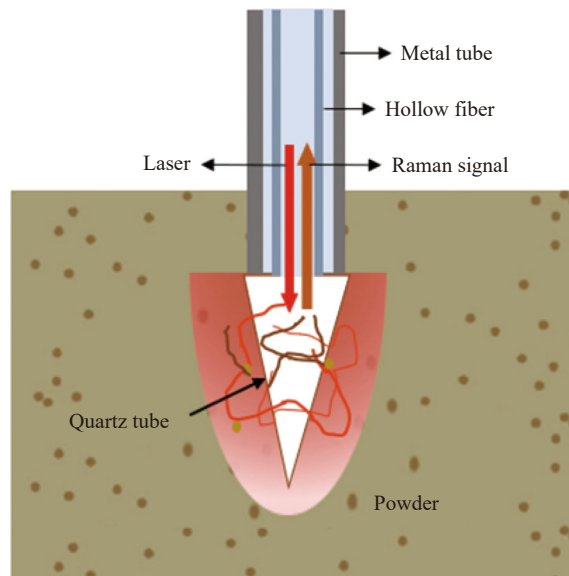
图 3 石英管增强拉曼光纤探头样品探测
