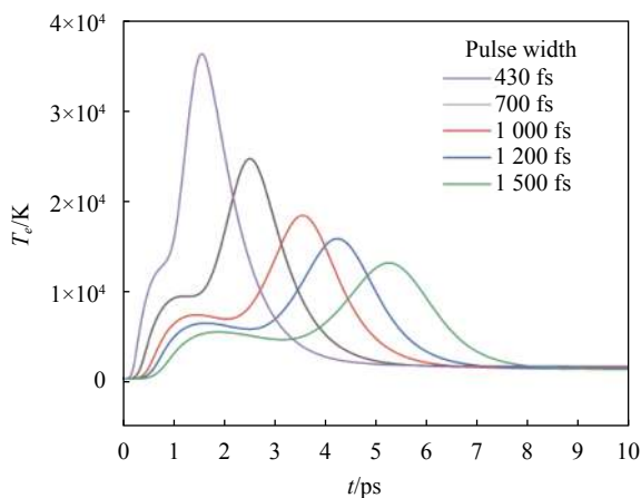
图 2 在脉宽分别为 430、700、1000、1200、1500 fs，能量密度为 0.35 J/cm 2 的激光辐照下电子温度随时间的变化 Fig.2 Variation of electron temperature with time under laser irradiation with pulse width of 430, 700, 1000, 1200, 1500 fs and energy density of 0.35 J/cm 2
