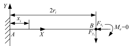
图 5 柔性铰链受力分析示意图
