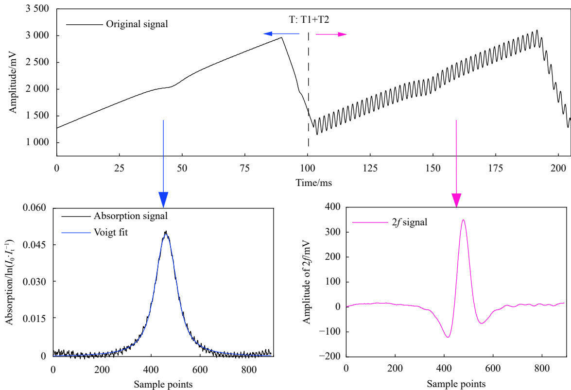
图 3 2.5% \text{CH}_4 的吸光度和二次谐波信号图
