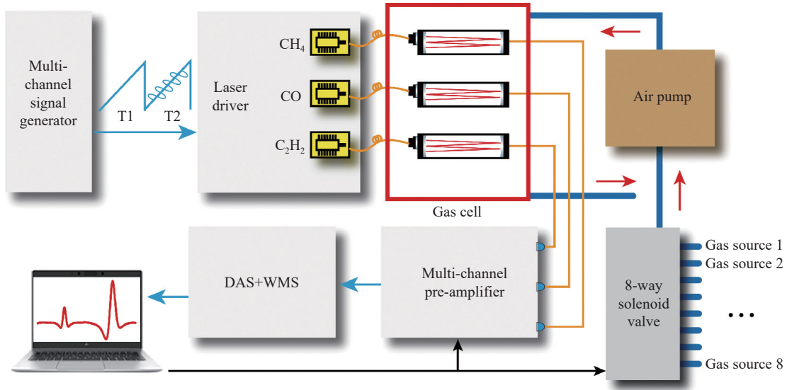
图 2 宽量程多气体检测系统方案示意图
