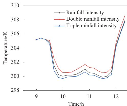
图 11 降雨阶段 CUBI 模型上面监测点温度对比图
