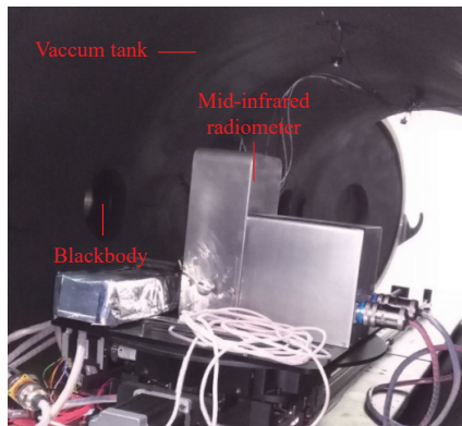
图 8 真空低温环境下中红外辐射计的标定现场
