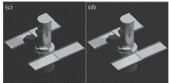
图 14 (a) 目标辐亮度图像; (b) 添加平台高频振动图像; (c) 添加光子噪声图像; (d) 高频振动及光子噪声共同作用图像
