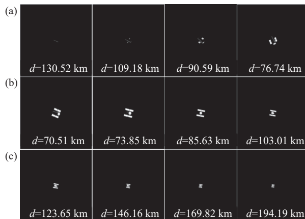
图 10 可见时间段内不同距离成像结果
