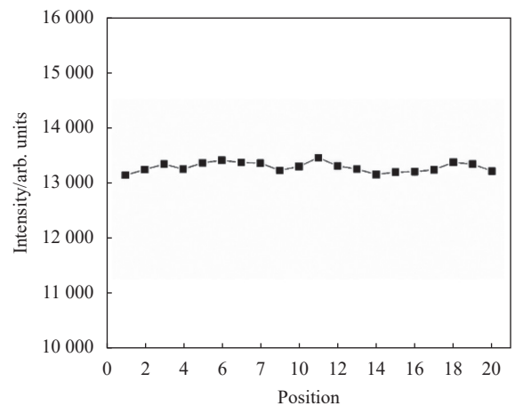
图 7 不同位置的谱线 Ga I 403.29 nm 的强度变化
