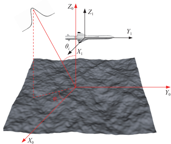
图 8 海面坐标系
