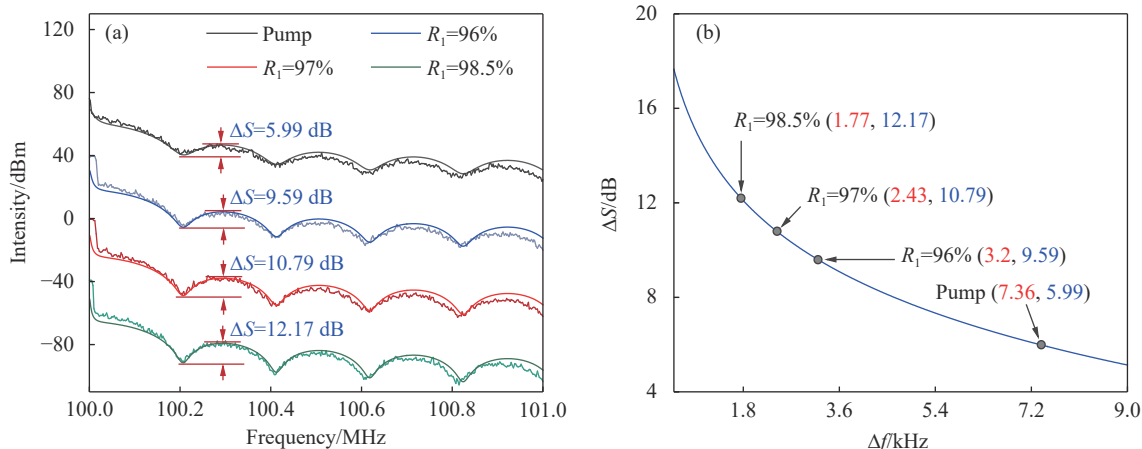
图 2 三组耦合镜反射率对应的 Stokes 线宽。(a) 延迟自外差测量得到的功率谱的幅度差; (b) 通过相干包络法计算的线宽和包络幅度差曲线
