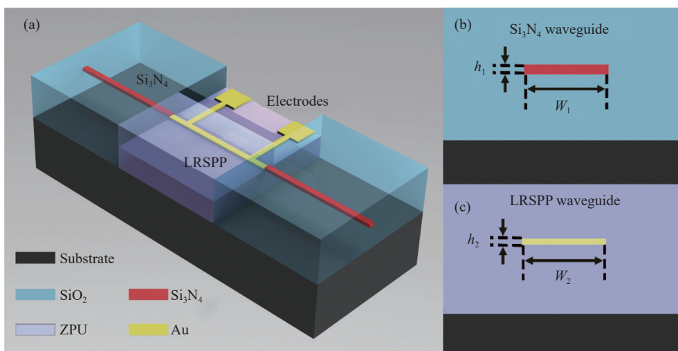
图 2 (a) 基于 \text{Si}_3\text{N}_4 和 LRSPP 波导的温度不敏感结构示意图; (b) \text{Si}_3\text{N}_4 波导横截面; (c) LRSPP 波导横截面
