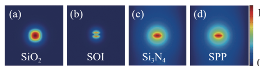
图 1 (a) \text{SiO}_2 波导的 TM 模; (b) SOI 波导的 TM 模; (c) \text{Si}_3\text{N}_4 波导的 TM 模; (d) LRSPP 波导的 TM 模
