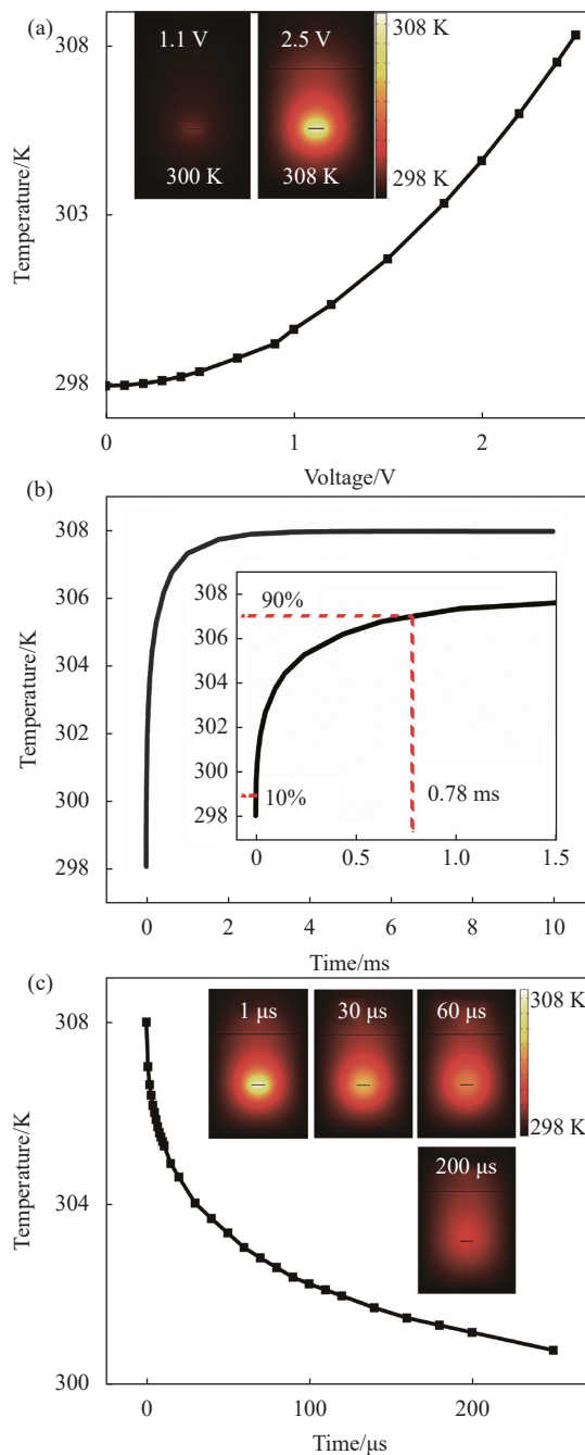
图 6 (a) LRSP 波导温度与施加电压的关系, 插图是不同电压下 LRSP 波导的温度场分布; (b) LRSP 波导的升温曲线, 插图是升温曲线局部放大图; (c) LRSP 波导的降温曲线, 插图是不同降温时间下 LRSP 波导的温度场分布
