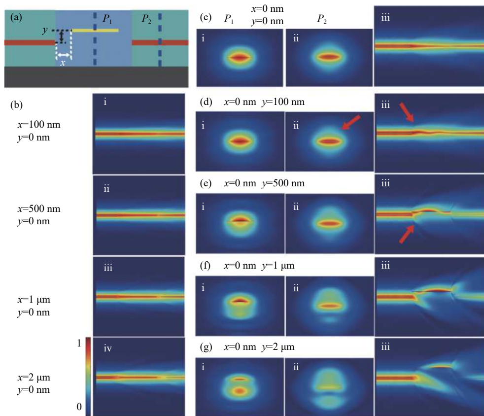
图 4 (a) \text{Si}_3\text{N}_4 波导和 LRSPP 波导在横向(x方向)和纵向(y方向)上的偏移;(b) \text{Si}_3\text{N}_4 波导和 LRSPP 波导横向偏移时的传输场;(c)-(g) \text{Si}_3\text{N}_4 波导和 LRSPP 波导在不同纵向偏移时的特性:(i) P_1 点的模式分布,(ii) P_2 的模式分布,(iii) 传输场
