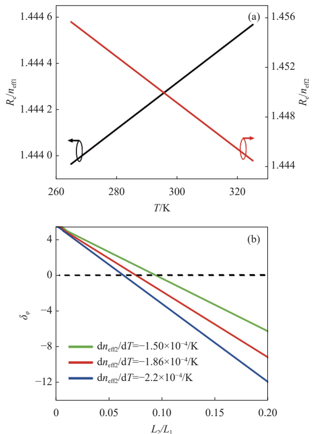
图 5 (a) Si 3 N 4 波导和 LRSP 波导模式有效折射率随温度的变化曲线; (b) 不同热光系数下, 相位变化与 Si 3 N 4 波导和 LRSP 波导长度比的关系
