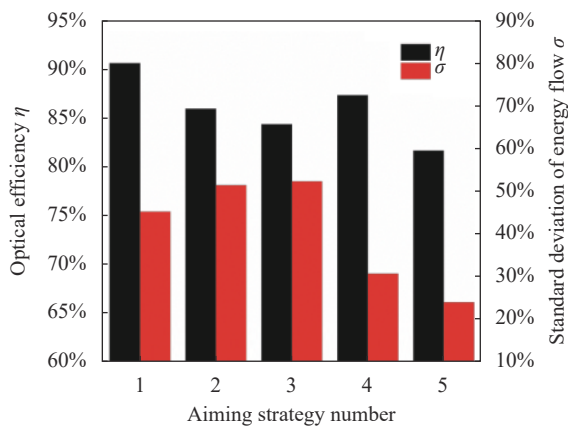
图 8 五种瞄准策略光学效率与能流标准差对比图
