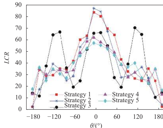
图 9 五种瞄准策略局部聚光比对比图
